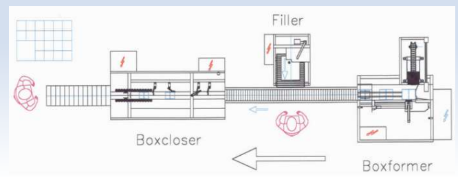
Aufstellungsvorschlag mit Eurofüller
