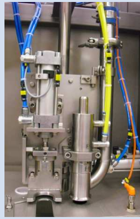
Füllkammer
